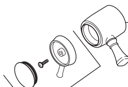
RP47198▲ Temperature Knob and Cover & Screw Perilla de la Temperatura y Cubierta y Tornillo Poignée de Réglage de Température et Vis
